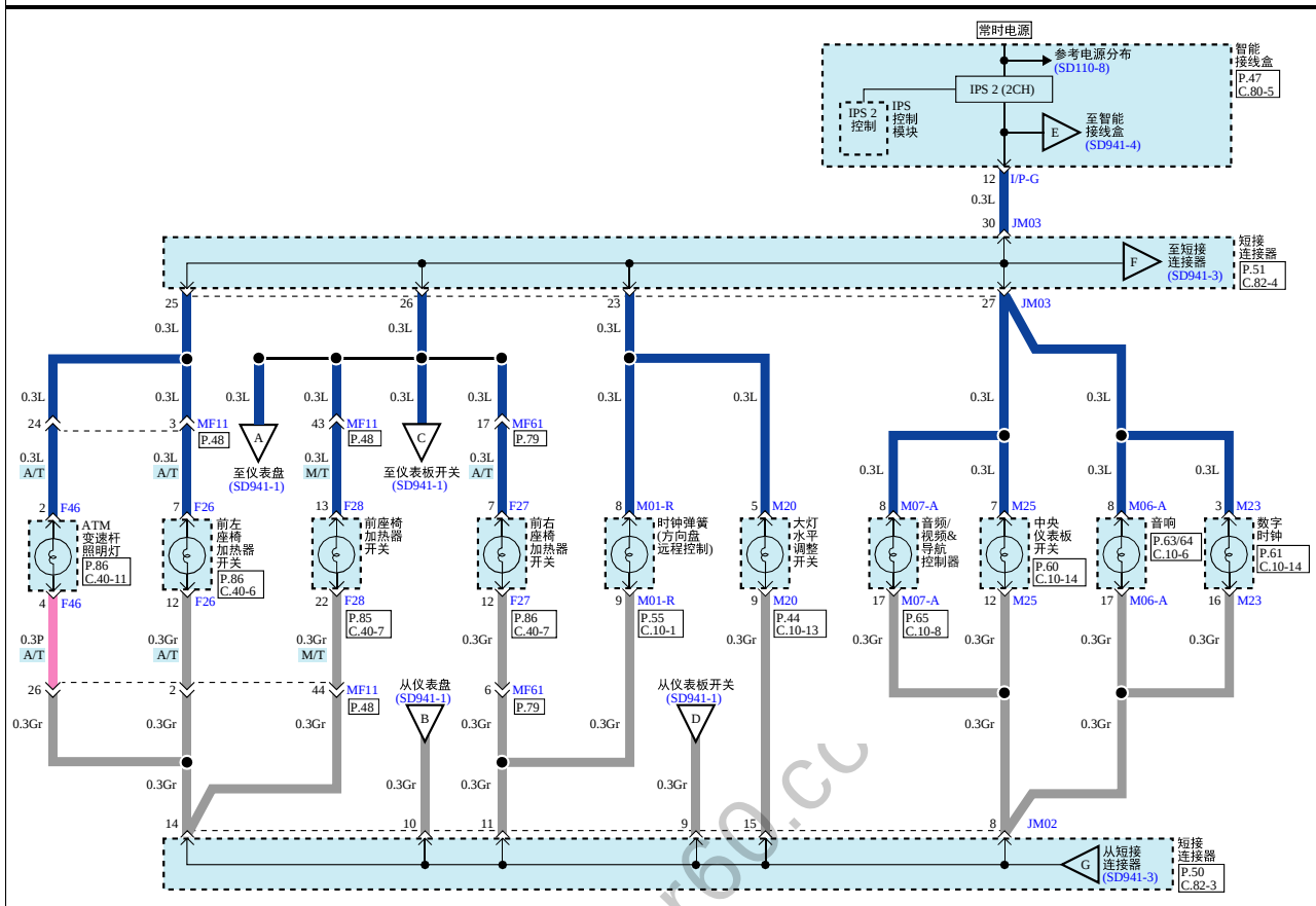
照明灯(2)
